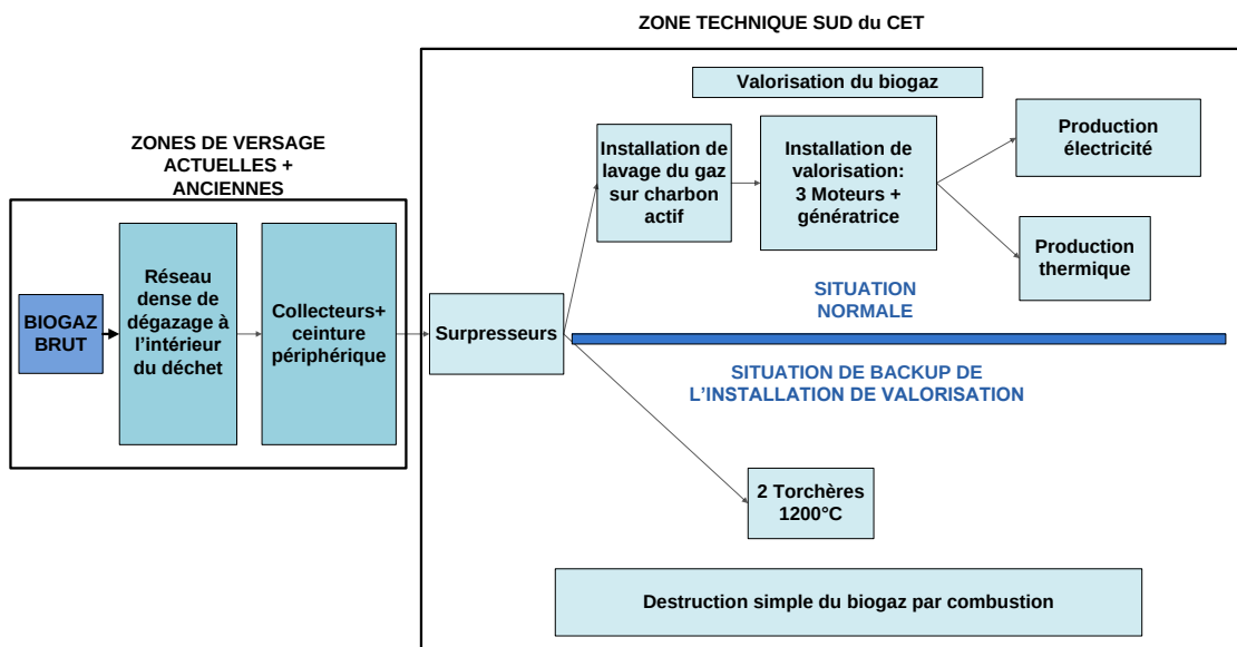
Figure 8 : Système de collecte et de gestion du biogaz (G)
