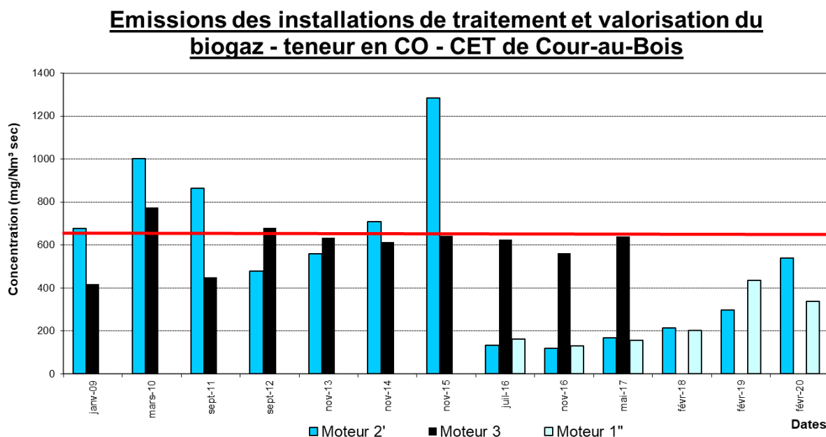
Figure 13 : Récapitulatif des mesures de concentration en CO (g) sur nos installations de valorisation du biogaz (g)
