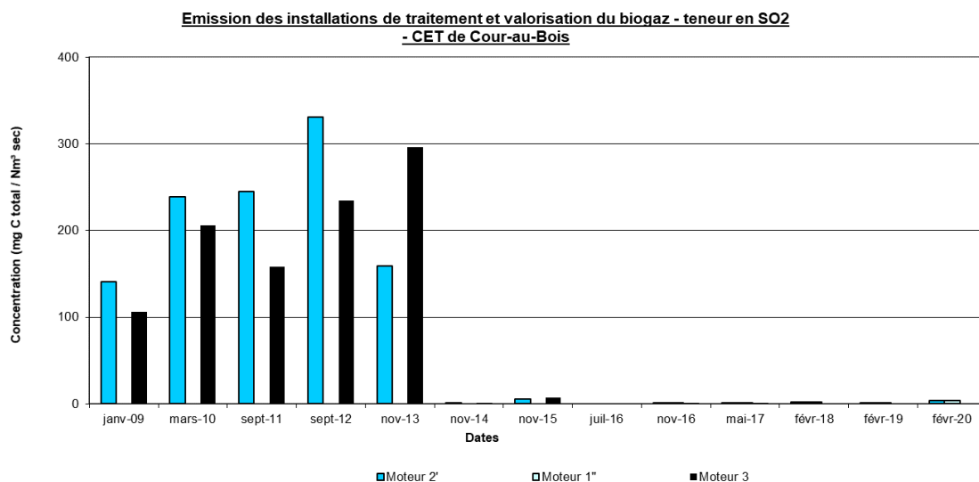
Figure 12 : Récapitulatif des mesures de concentration en SO 2 (g) sur nos installations de valorisation du biogaz (g)
