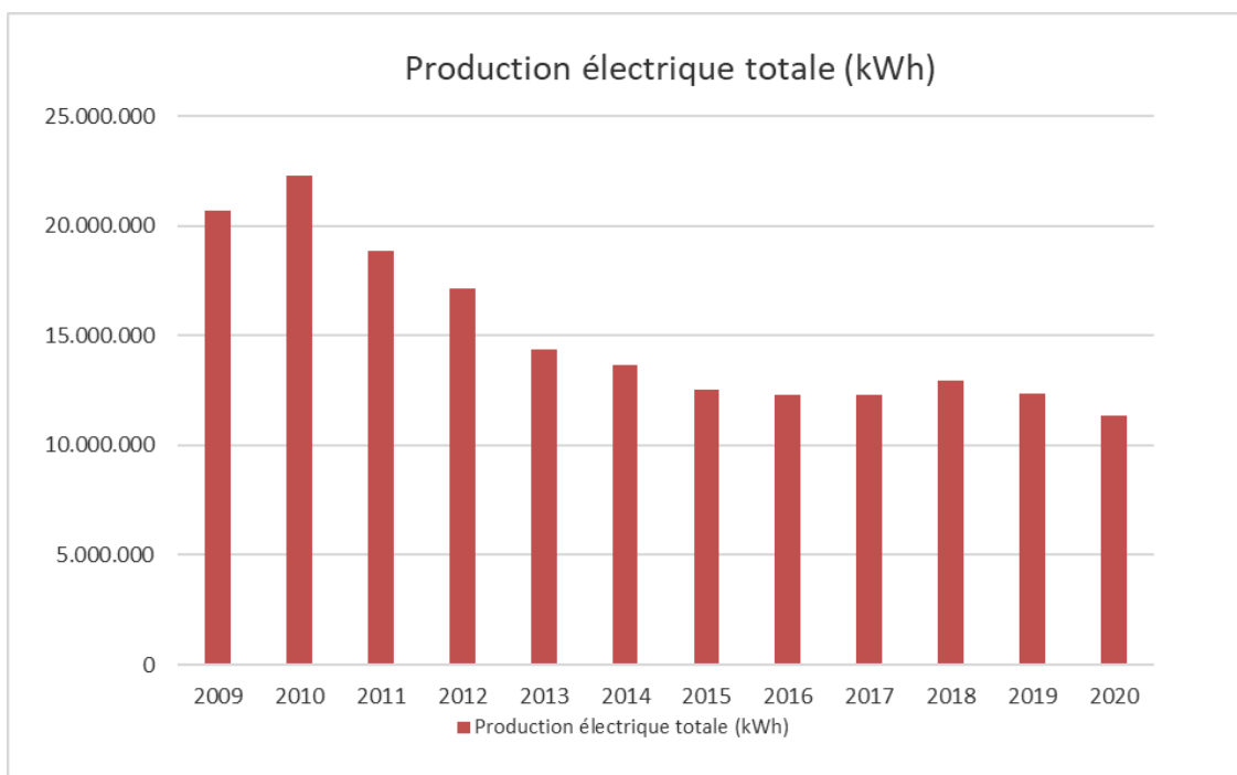
Figure 14 : Evolution de la production électrique annuelle de nos installations de valorisation du biogaz (9)
