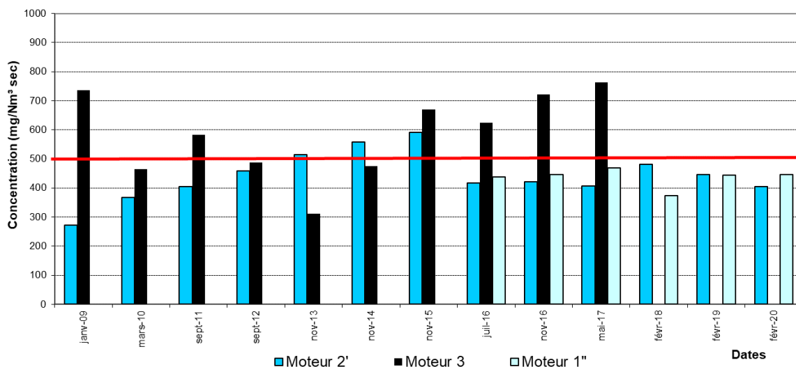
Figure 11 : Récapitulatif des mesures de concentration en NOx (g) sur nos installations de valorisation du biogaz (g)
